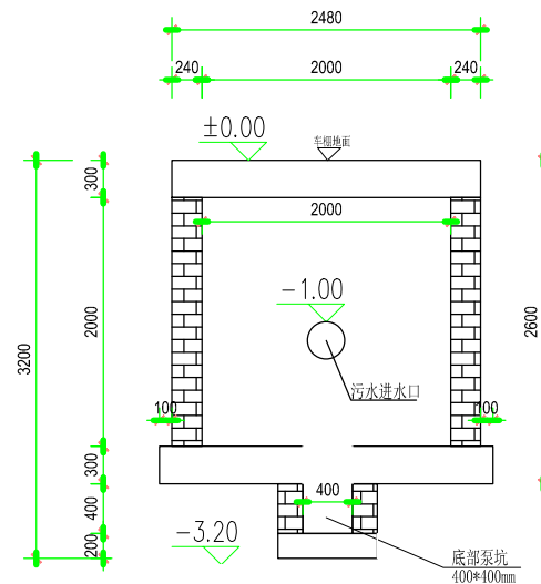
新建集水井立面图
