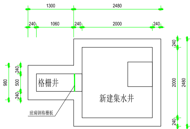
新建集水井平面图
